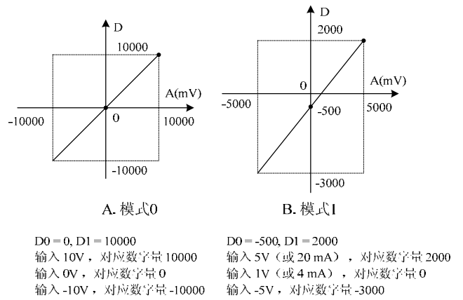
图 3-3 特性更改举例
