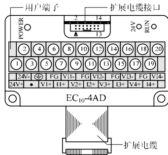
图 1-2 模块接口端子图
