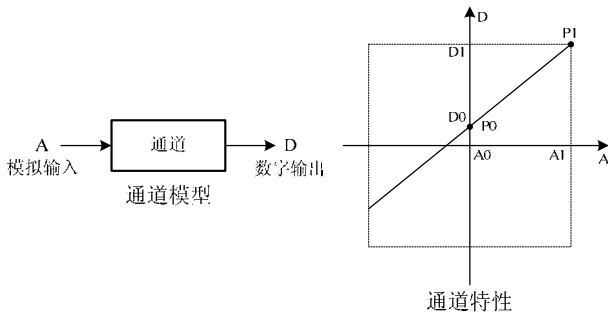
图 3-1 EC10-4AD 的通道特性示意图
