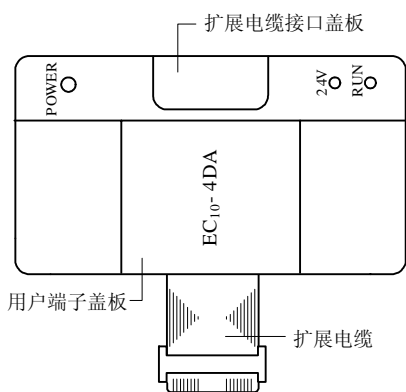
图 1-1 模块接口外观图
