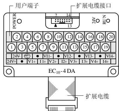
图 1-2 模块接口端子图
