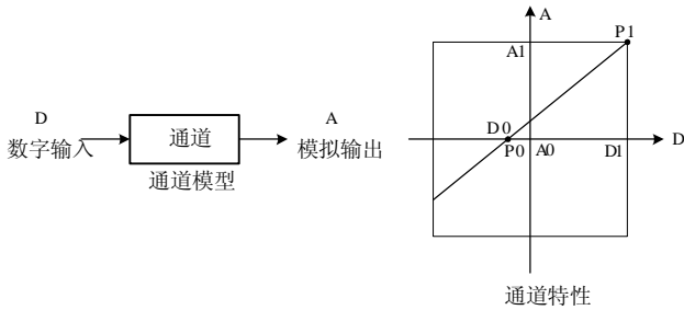
图 3-1 EC10-4DA 的通道特性示意图
