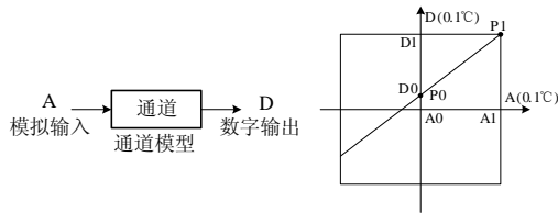
图 3-1 EC10-4TC 的通道特性示意图
