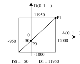
图 3-3 特性更改举例
