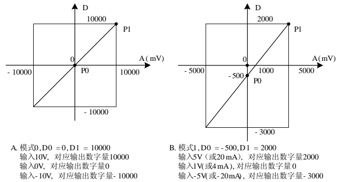
图 3-3 输入通道特性更改举例
