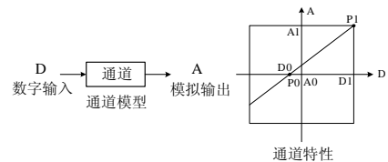
图 3-4 EC10-5AM 的输出通道特性示意图
