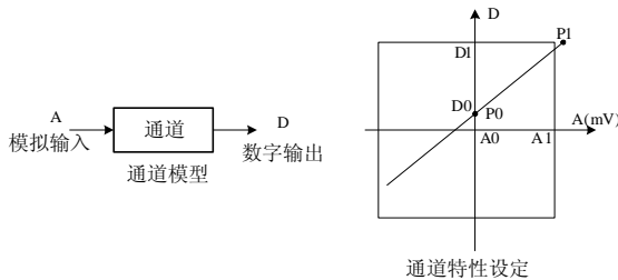
图 3-1 EC10-5AM 的输入通道特性示意图
